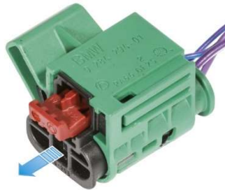
Service Disconnect ziehen
