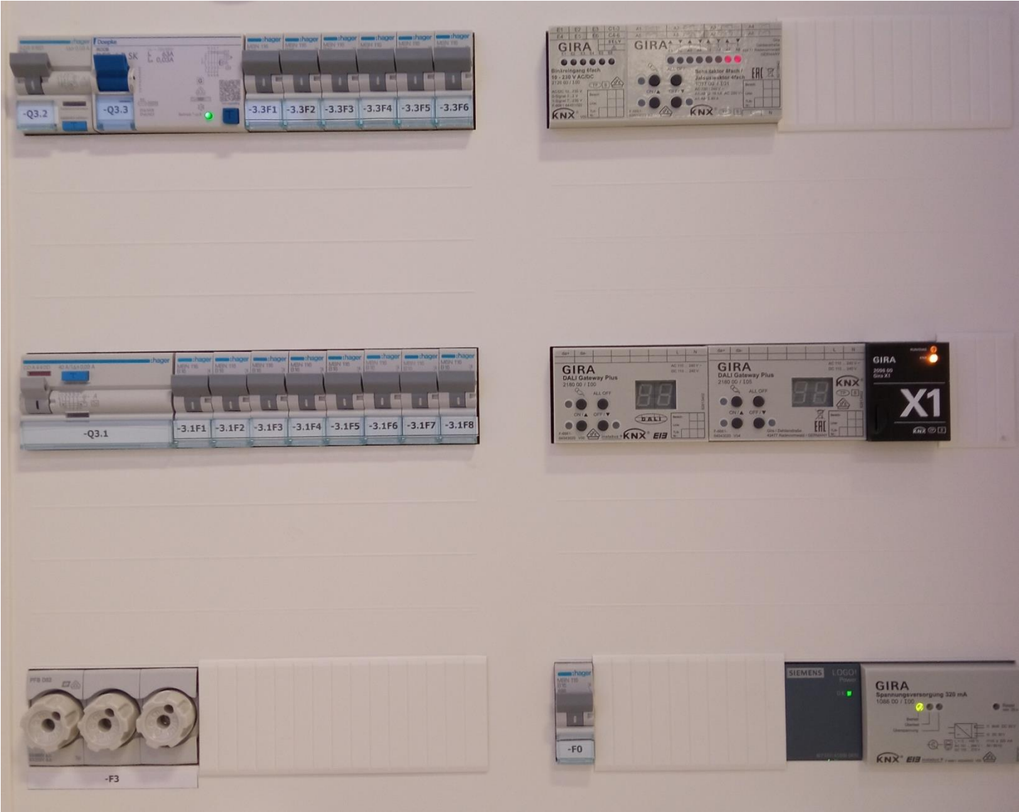
Bild 1: Unterverteilung Feld rechts unten
